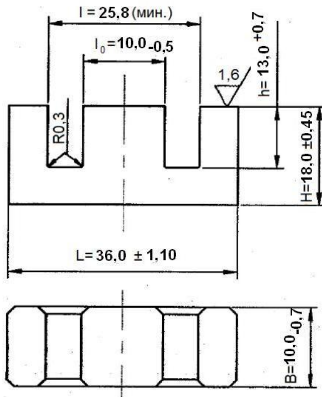
Рис. 1. Сердечник EE36A
