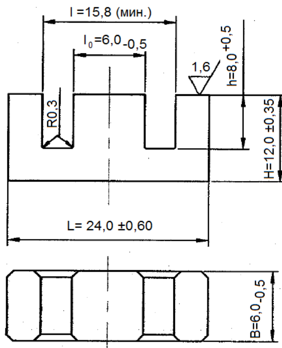
Рис. 1. Сердечник EE24D
