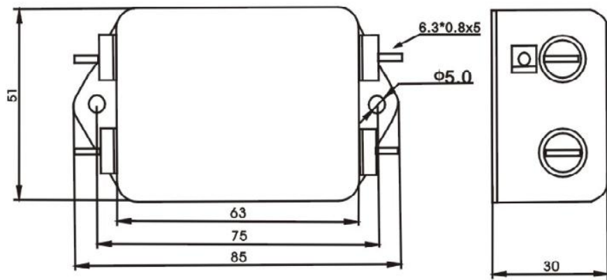
DBA4-10A
