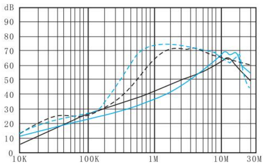
DBA4-20A/DBA4-10A
