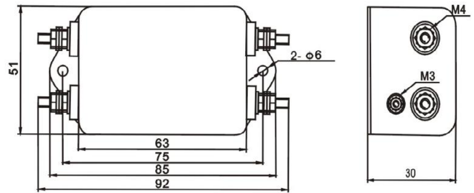
DBA4-20A
