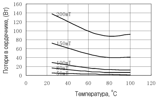
Потери на частоте 100 кГц
