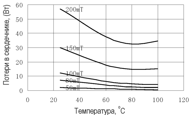
Потери на частоте 50 кГц
